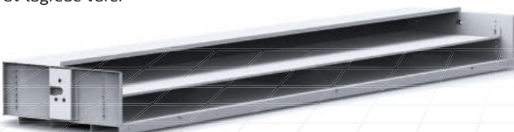
Lastbærer med selvstøttende mellomliggende hylle for lagring av store, flate varer
